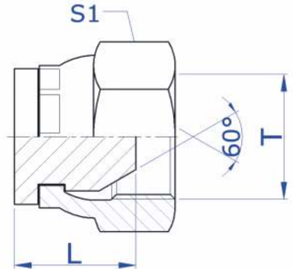
DIŞİ KÖR TAPA FEMALE BLANKING PLUG
