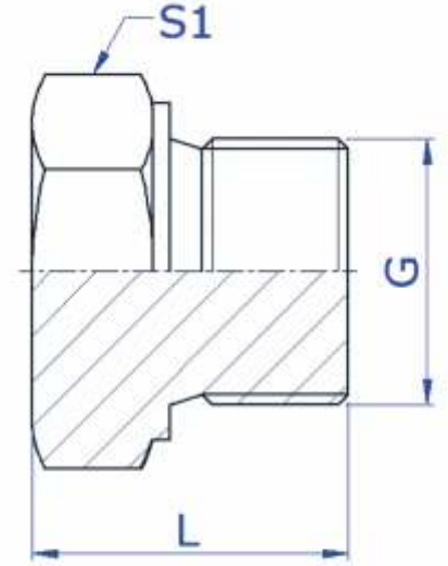
ERKEK KÖR TAPA MALE BLANKING PLUG
